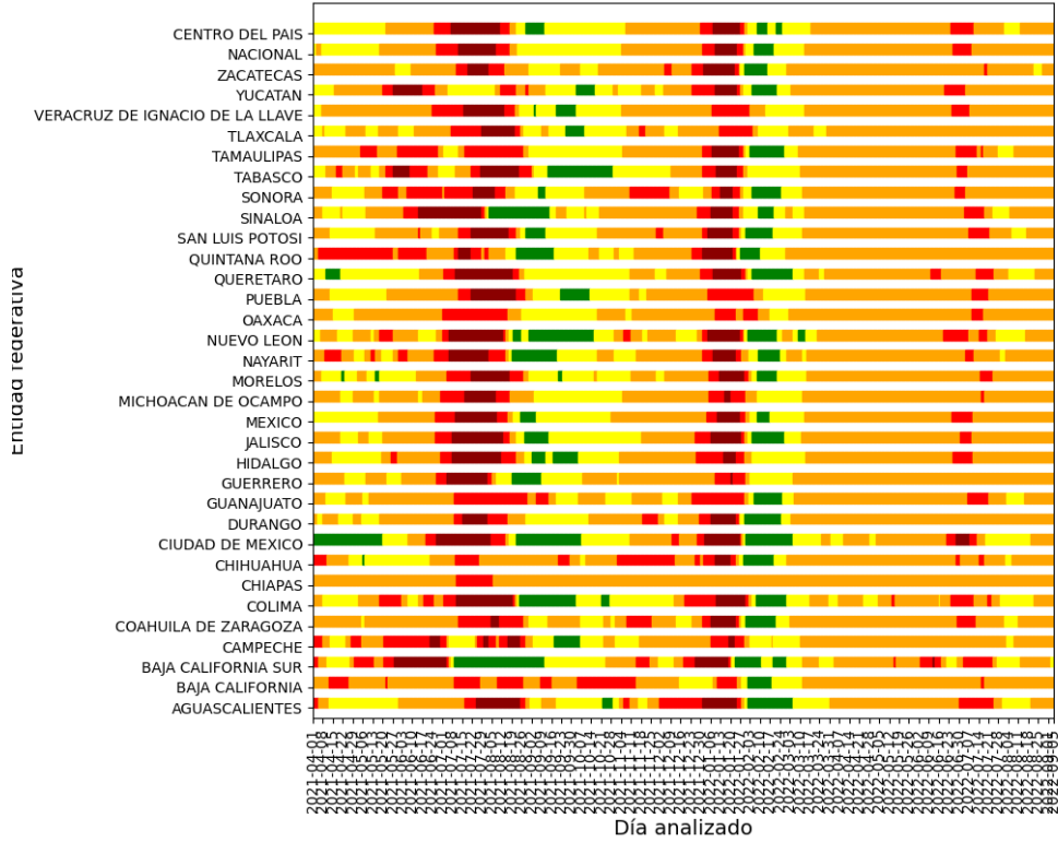
Cálculo de la tendencia por estado: 2022-09-05 (D=0, S=0.0050)
