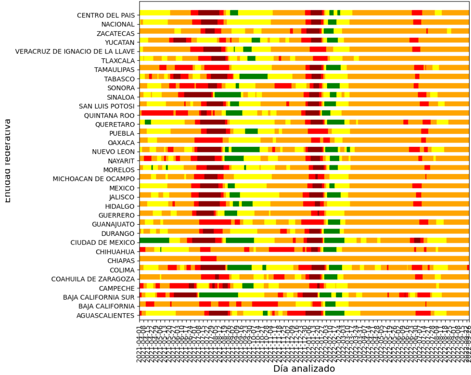
Cálculo de la tendencia por estado: 2022-09-26 (D=0, S=0.0050)
