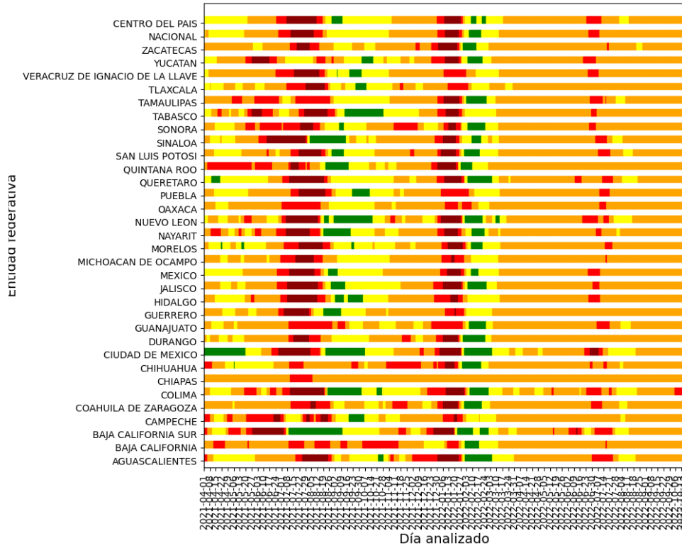
Cálculo de la tendencia por estado: 2022-10-17 (D=0, S=0.0050)
