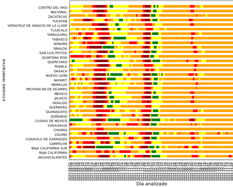
Cálculo de la tendencia por estado: 2022-12-05 (D=0, S=0.0050)
