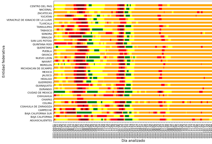
Cálculo de la tendencia por estado: 2023-02-13 (D=0, S=0.0050)
