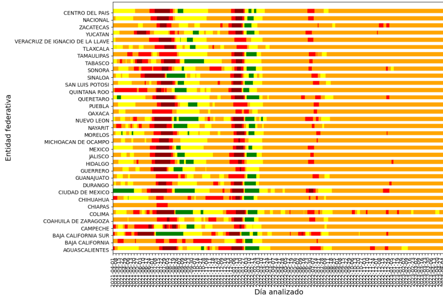
Cálculo de la tendencia por estado: 2023-05-08 (D=0, S=0.0050)
